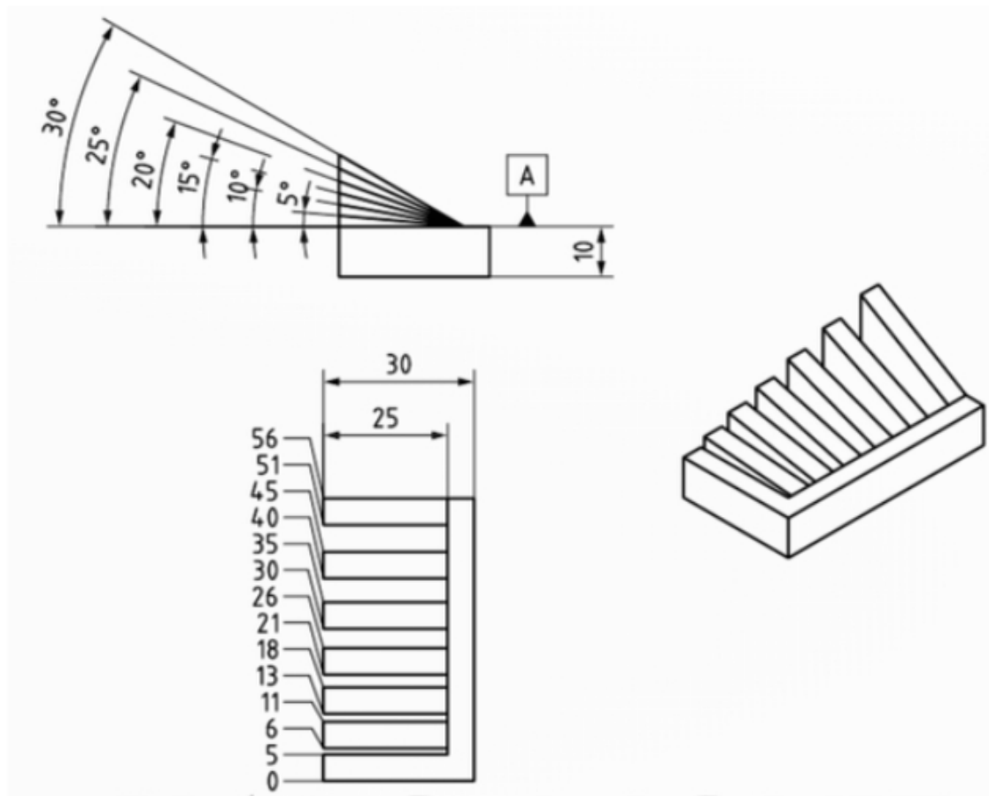
그림 9 — 굽은 분해능 슬롯 경사 형상의 도면
