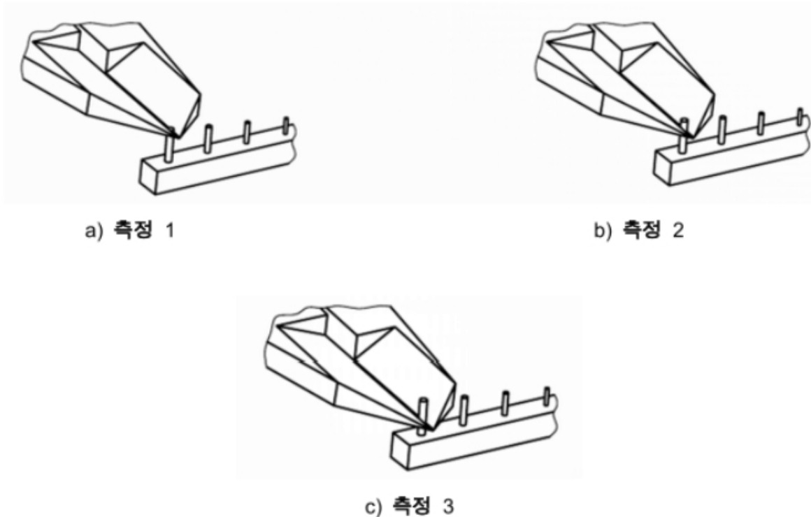
그림 C.3 - 업스탠드 측정
