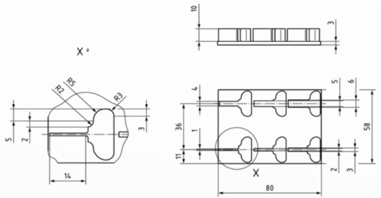
그림 7 — 굵은 분해능 리브 형상의 도면
